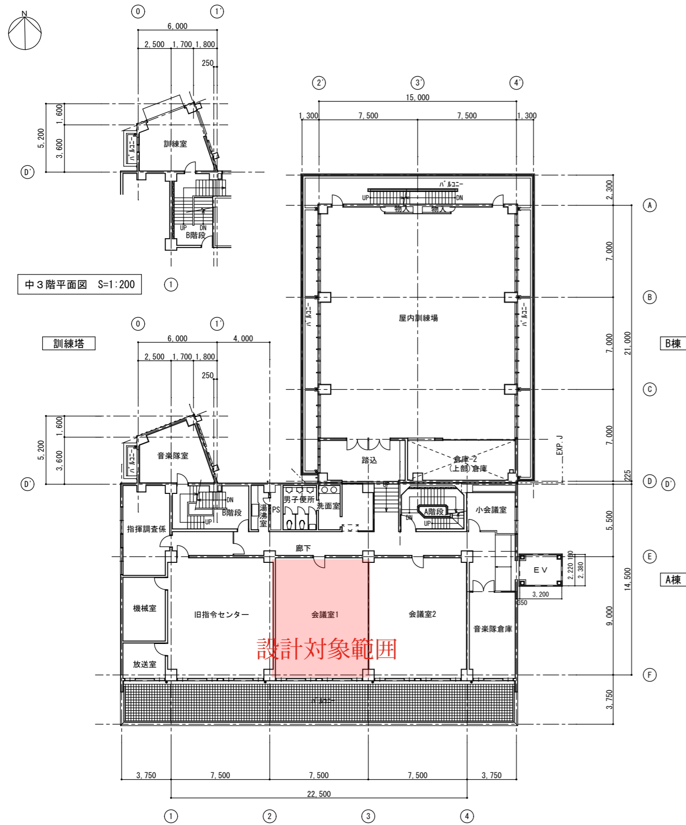
3階平面図
