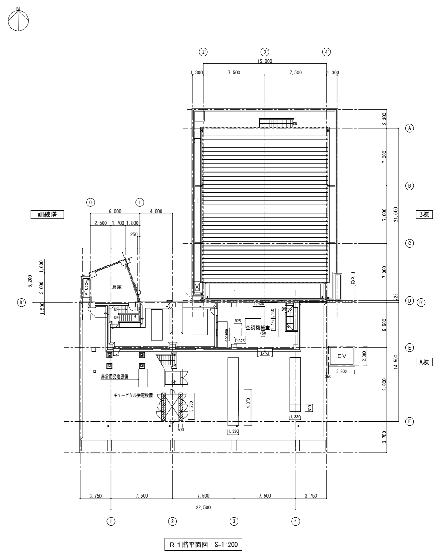
R 1階平面図
